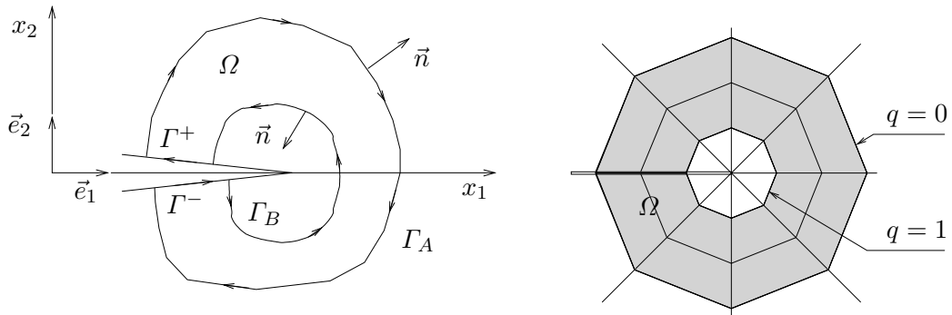
Fig. 11.13 : J-integral domain.
