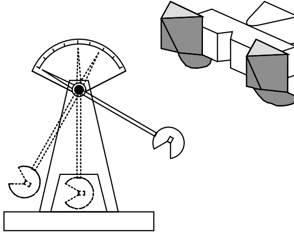
Fig. 2.6 : Charpy V-notch test.
